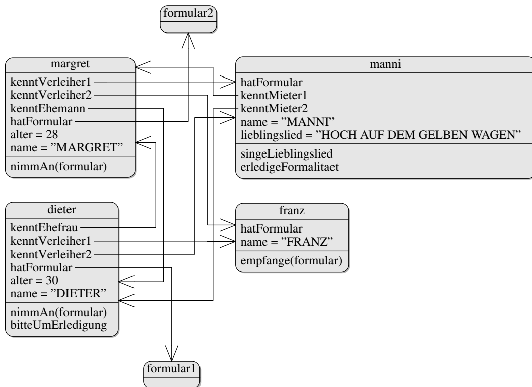
Abbildung 2: Ein Objektdiagramm
